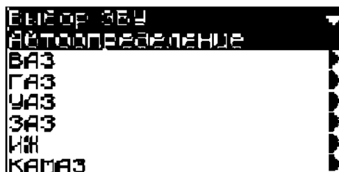
Рис. 2 Главное меню
