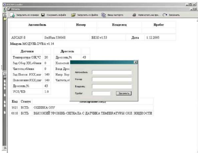
Рис. 31 Окно ПЕЧАТЬ
