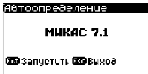
Рис. 8 Автоопределение модуля
